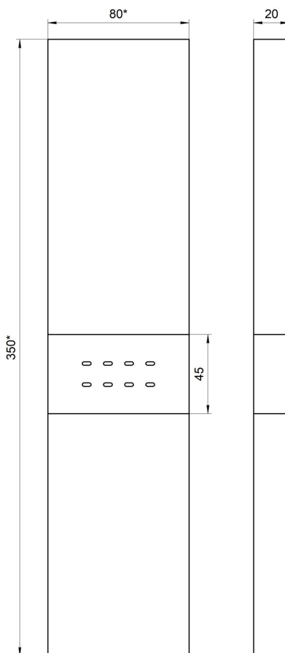
Рис.1 Внешний вид «Указатель лифтовой» НШЕК.468232.203
